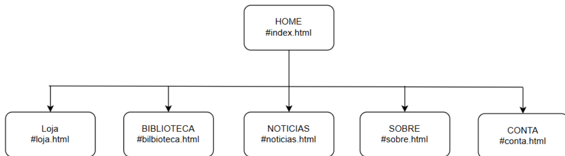
Fig3: Diagrama de estrutura hierárquica e navegação das secções da plataforma
