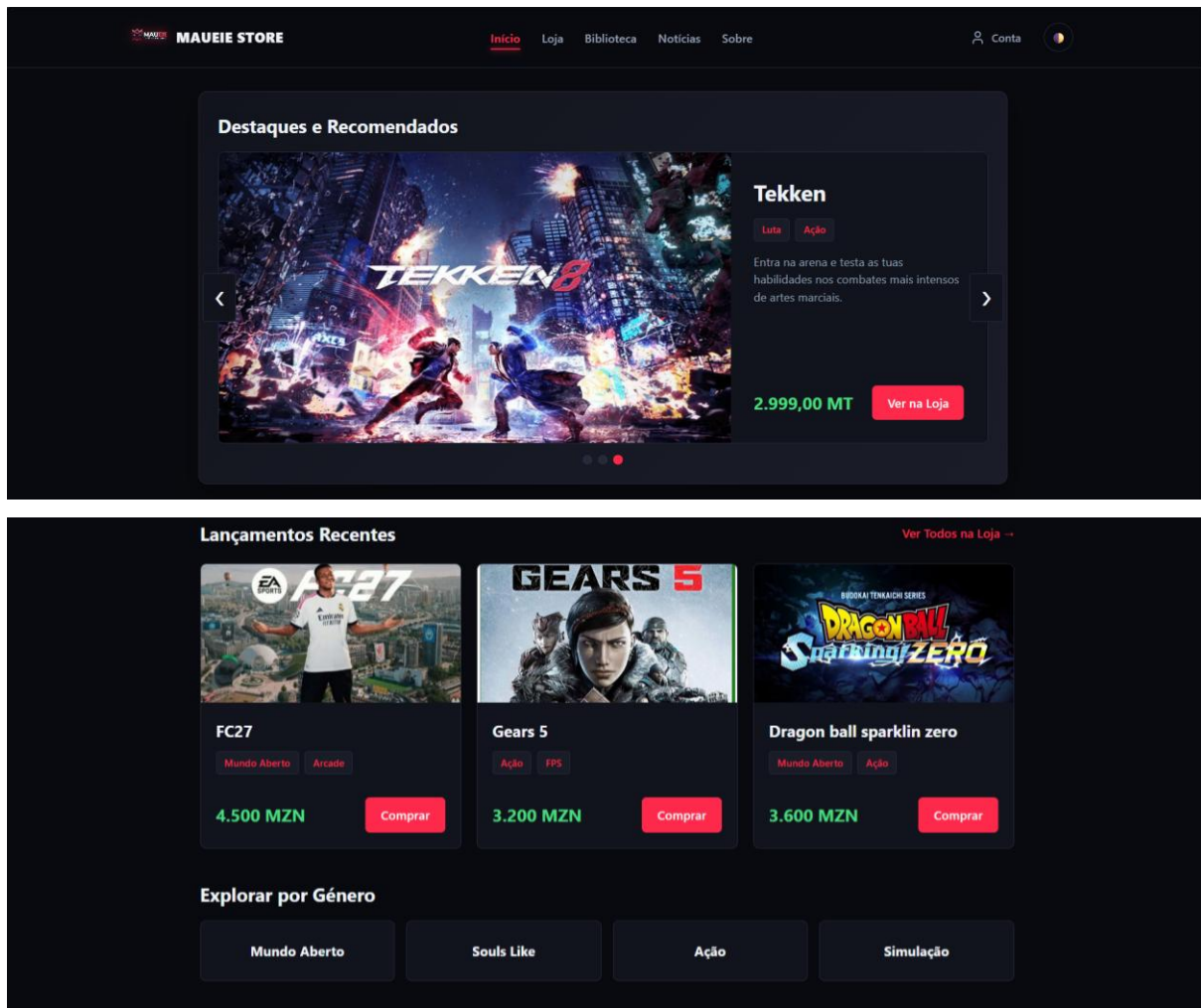
Fig5: Representação do esquema estrutural do Wireframe (layout funcional da Home):
